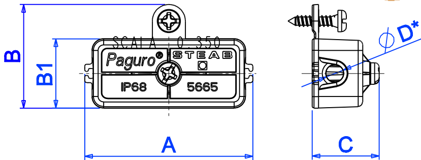
Esempio di montaggio Assembly's example
